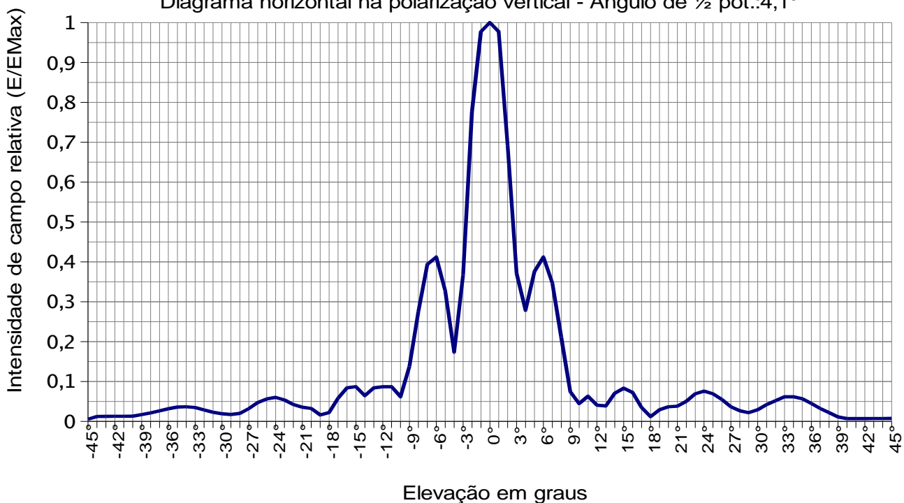
Antena parabólica 55cm para enlace na frequência de 7 GHz Diagrama horizontal na polarização vertical - Ângulo de ½ pot.:4,1°
