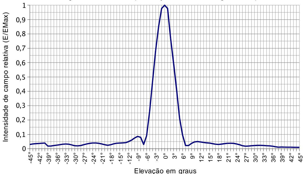
Antena parabólica 55cm para enlace na frequência de 7 GHz Diagrama horizontal na polarização horizontal - Ângulo de ½ pot.:5°
