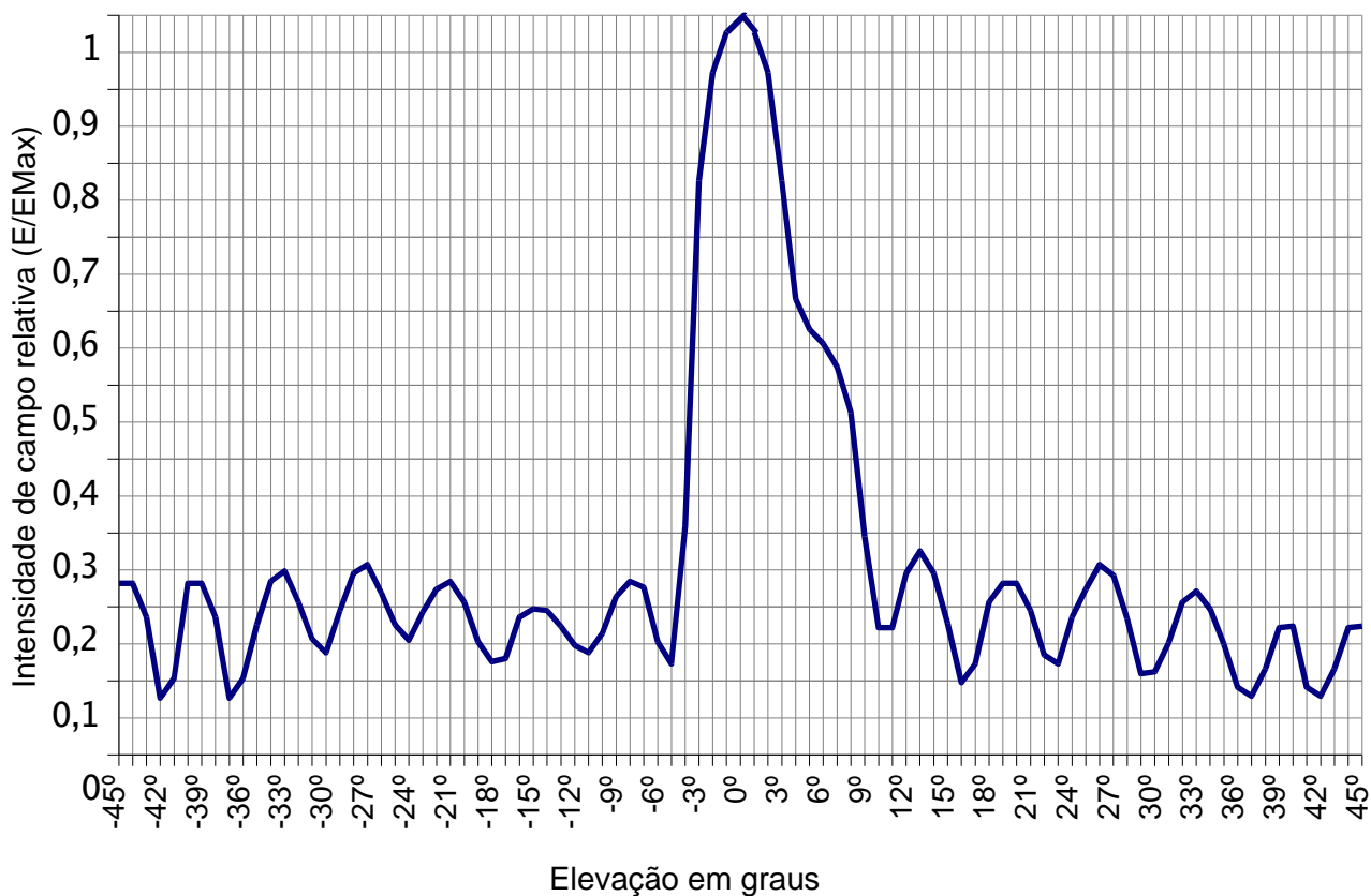
Painel setorial para WLL Elevação para 15 dBi
