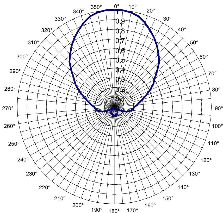
Antena Setorial tipo Painel Diagrama horizontal - Ângulo de ½ pot.: 90°
